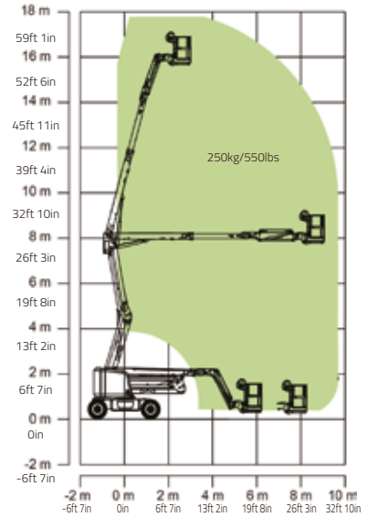
Hareket Aralığı ZA16JERT/ZA16JERT-Li
