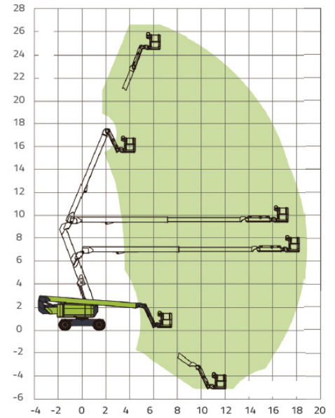
ZA24J Çalışma Diyagramı
